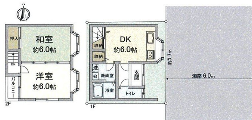
【間取り図】
