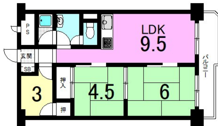
【間取り図】
