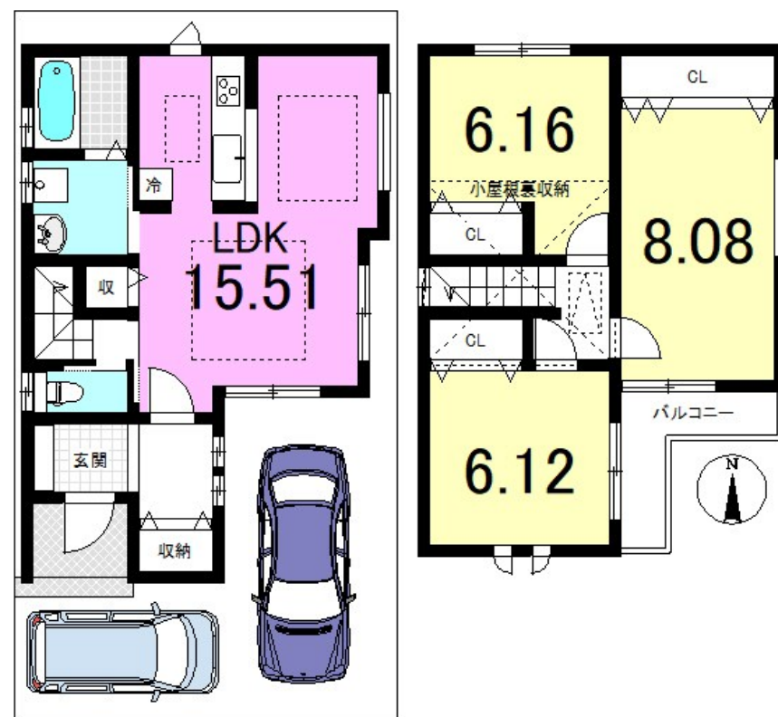
【間取り図】
