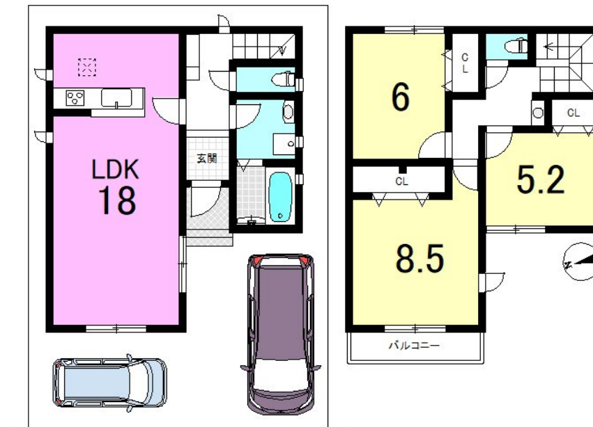
【間取り図】
