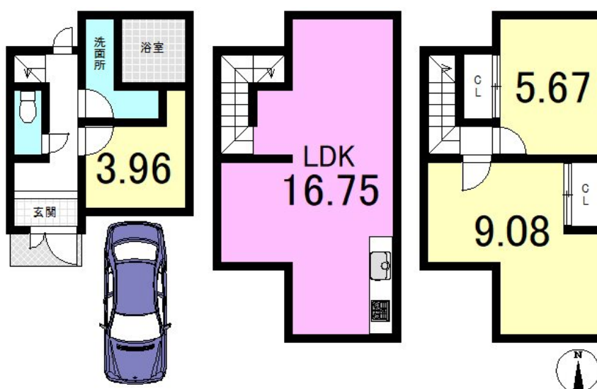
【間取り図】
